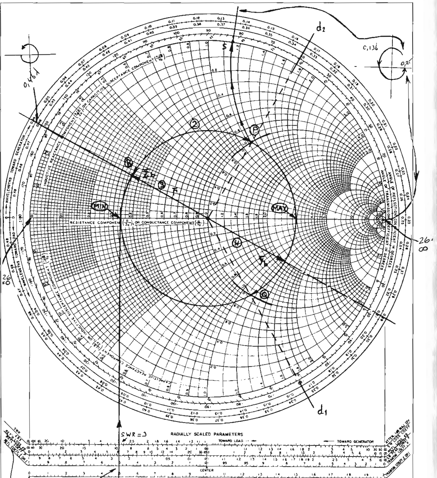
Uitgewerkt voorbeeld Smith-Chart
